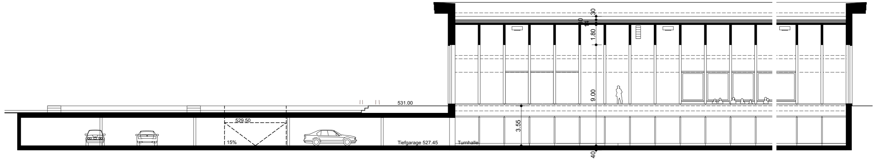
LS - Einstellhalle / Sporthalle
